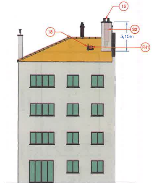
FACADE EST
