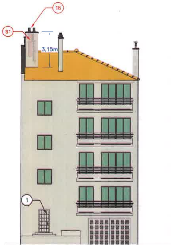
FACADE OUEST
